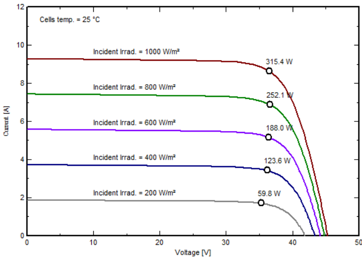
PV module: Waaree, WS-315_4BB-40-01
