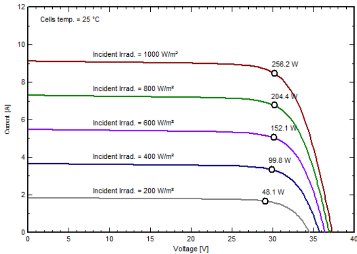
PV module: Waaree, WS-255
