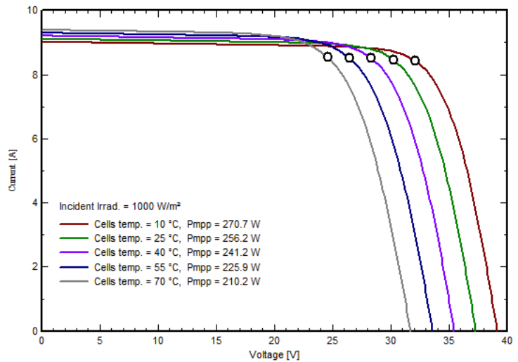
PV module: Waaree, WS-255
