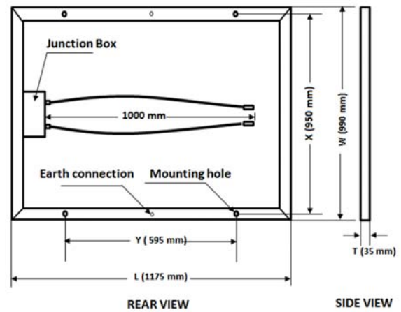
PV module: Waaree, WS-150 / 24V
