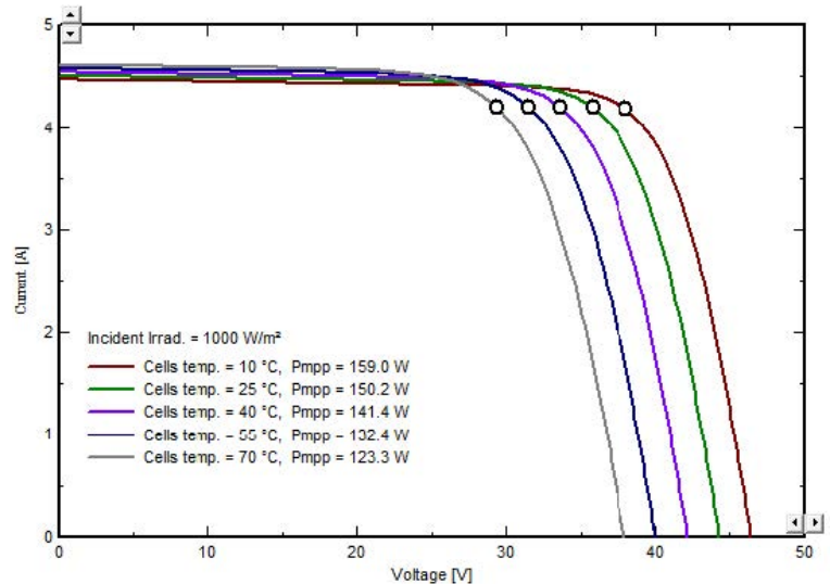
PV module: Waaree, WS-150 / 24V
