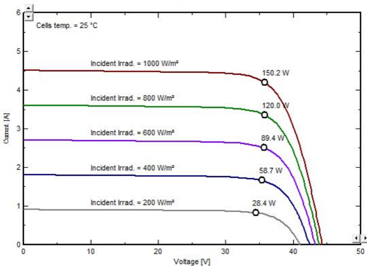
PV module: Waaree, WS-150 / 24V
